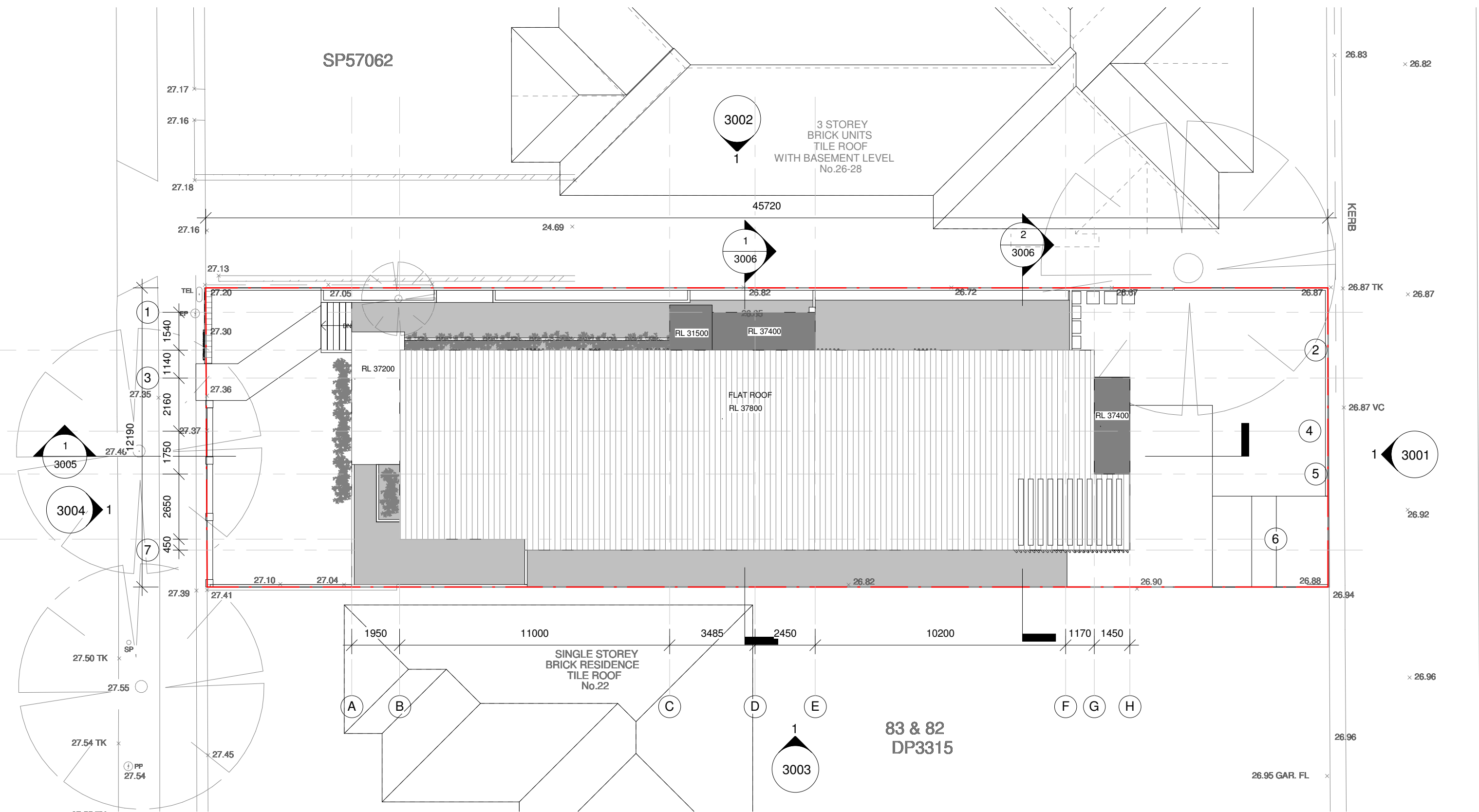
1 ROOF PLAN 1 : 150
